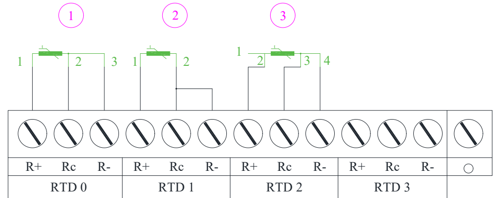
热电阻接线示意图
